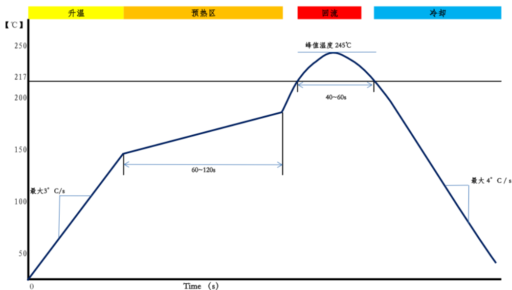
图 8-1 MXT901D 推荐炉温曲线
