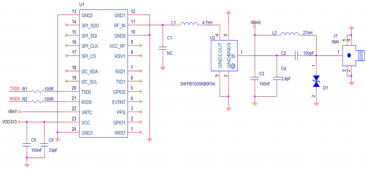
图 7-1 MXT901D 参考设计
