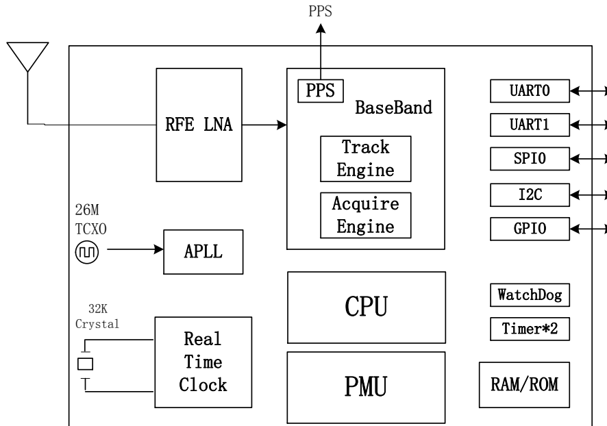
图 1-2 模块框图
