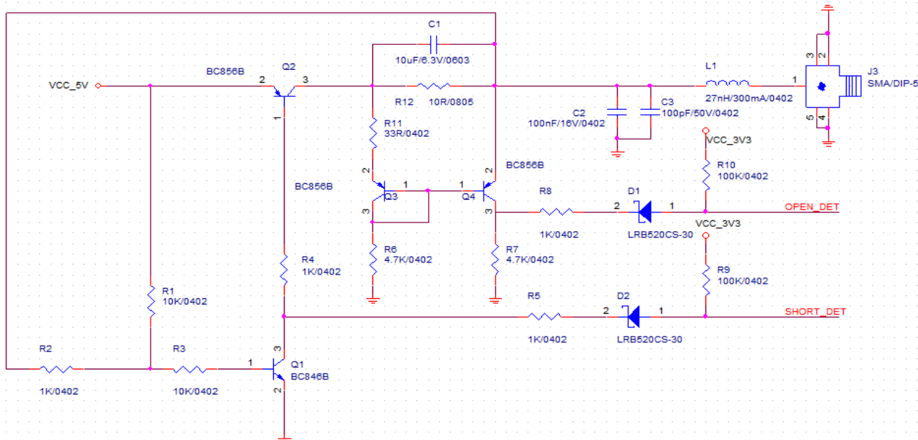
图 7-3 MXT901D 天线检测参考电路
