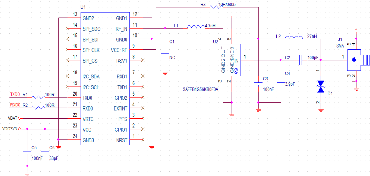
图 7-2 MXT901D 模块 VCC_RF 馈电参考设计
