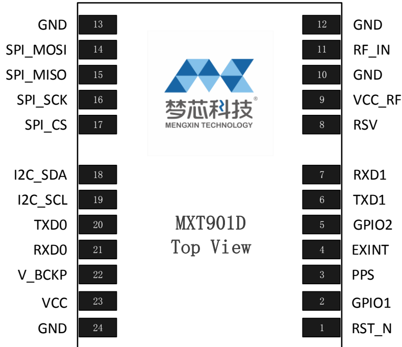
图 2-1 PIN 脚示意图
